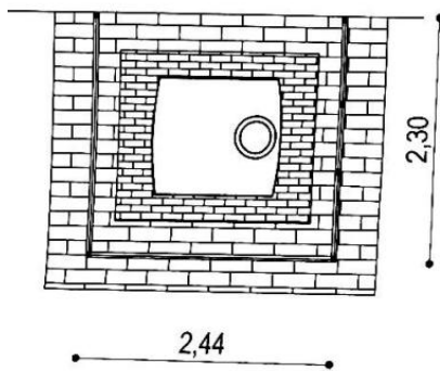
PIANTA DEPOSITO IDRICO
