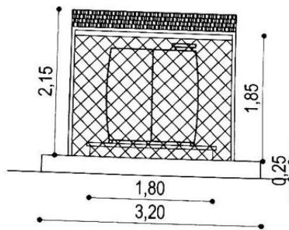
FRONTE DEPOSITO IDRICO
