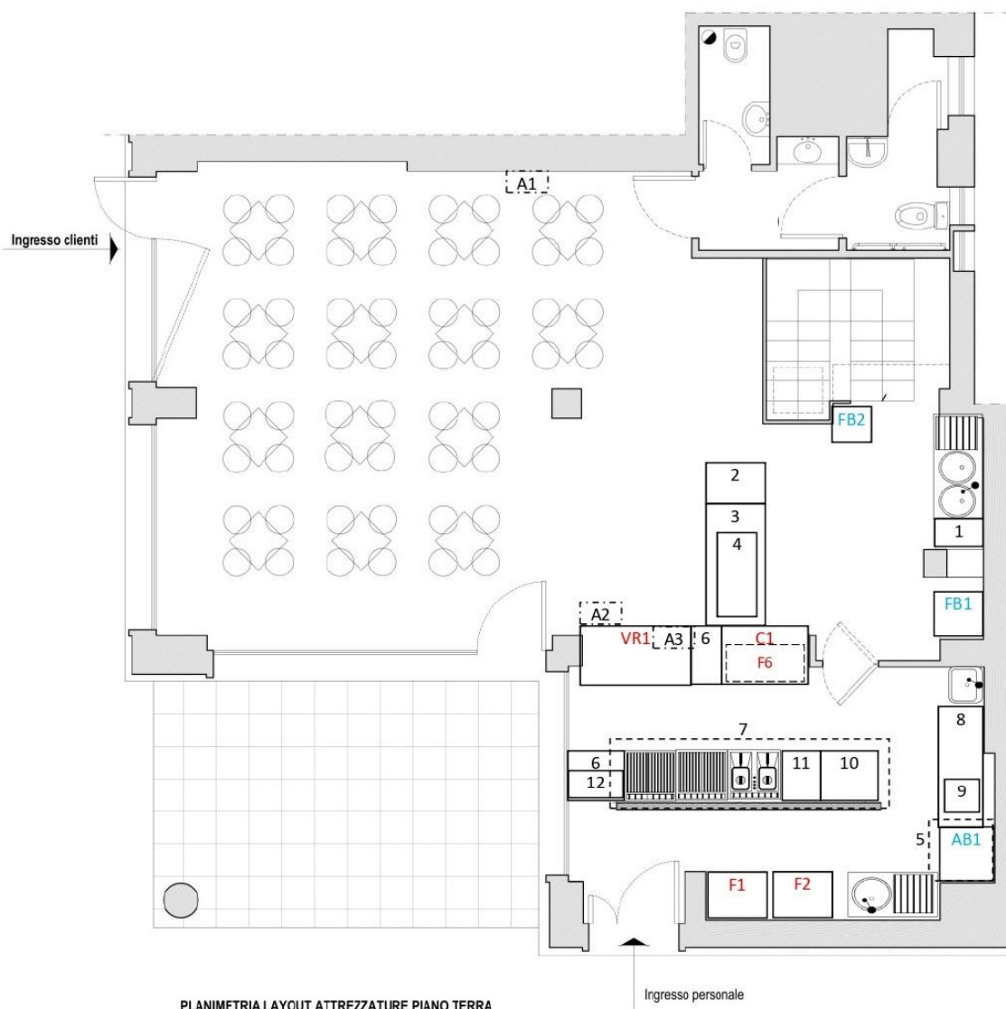
PLANIMETRIA LAYOUT ATTREZZATURE PIANO TERRA
