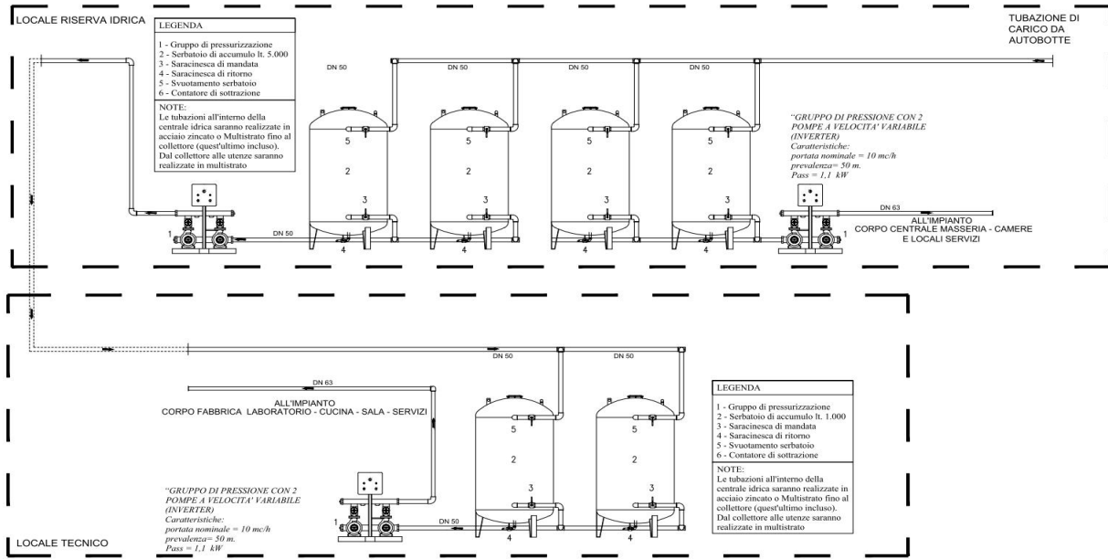
SCHEMA DI CENTRALE IDRICA
