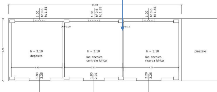
CORPO DI FABBRICA - DEPOSITO 2 SC. 1:100
